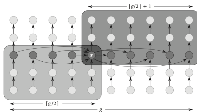
Figura 9.3 Le relazioni tra gli elementi di A (rappresentati da cerchi) subito dopo la riga 17 dell'algoritmo di selezione SELECT. Ci sono g = (r - p + 1)/5 cinque di elementi, ognuna delle quali occupa una colonna. Per esempio, la colonna più a sinistra contiene gli elementi A[p], A[p + g], A[p + 2g], A[p + 3g], A[p + 4g] e la colonna successiva contiene A[p + 1], A[p + g + 1], A[p + 2g + 1], A[p + 3g + 1], A[p + 4g + 1] . Le mediane dei gruppi sono i cerchi scuri e il pivot x è indicato con una etichetta. Le frecce vanno dagli elementi più piccoli a quelli più grandi. Gli elementi su sfondo grigio in basso a sinistra sono tutti minori o uguali a x e non possono cadere nella sezione alta della partizione fatta intorno a x . Gli elementi su sfondo grigio in alto a destra sono maggiori o uguali a x e non possono cadere nella sezione bassa della partizione fatta intorno a x . Il pivot x appartiene a entrambe le regioni con sfondo grigio ed è mostrato su uno sfondo più scuro. Gli elementi su sfondo bianco potrebbero trovarsi in entrambe le sezioni della partizione.
